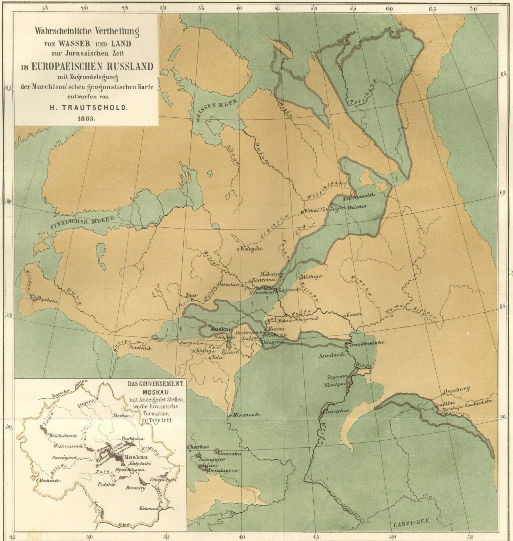
Die mit Lila umzogenen Theile des Meeres stellen Jurassischen Meeresboden dar, der grösstentheils zur Kreidezeit schon trocken gelegt war (Ausnahmen sind einige Theile des Gouvernem. Moskau, Ssaratow u. s. v., wo Kreideablagerungen den Jura bedecken), die mit ? bezeichneten Stellen des Meeres deuten an, dass hier noch kein Jura gefunden ist, dass aber das Dasein von Verbindung zwischen den verschiedenen Meerestheilen nicht unwahrscheinlich ist.
